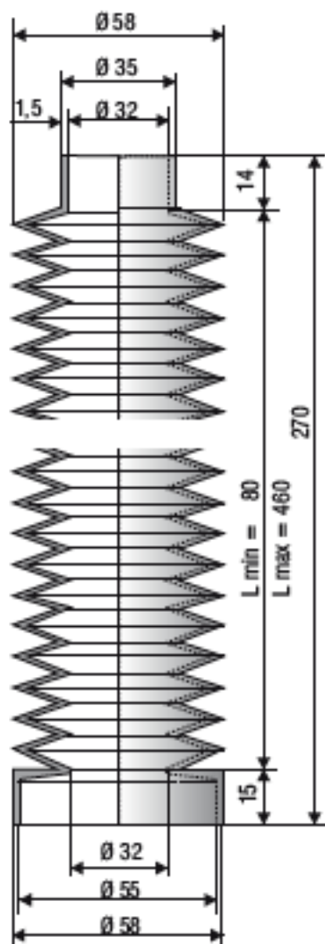
F 2029 NBR
