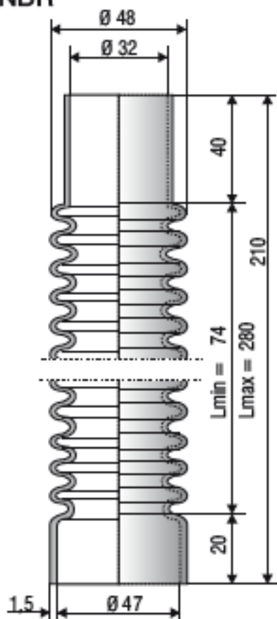
F 1115 NBR
