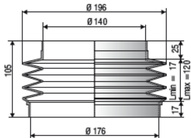
F 1110 NBR
