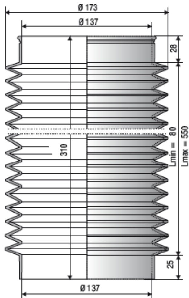
F 1181 NBR
