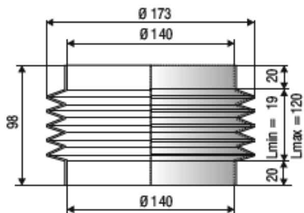
F 1046 NBR
