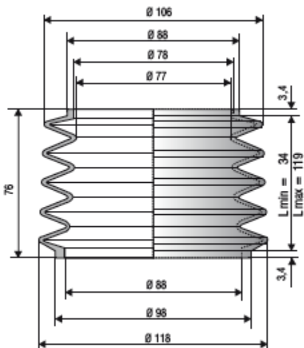
F 2012 NBR
