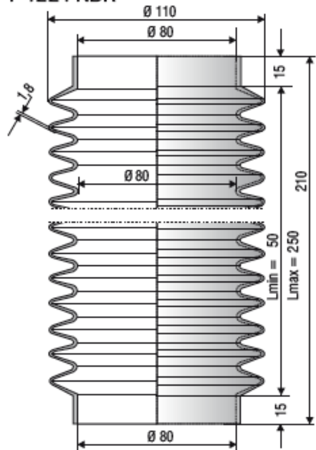
F 1224 NBR
