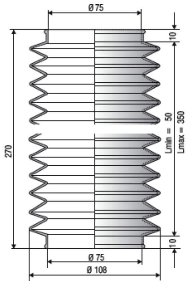
F 1224 NBR
